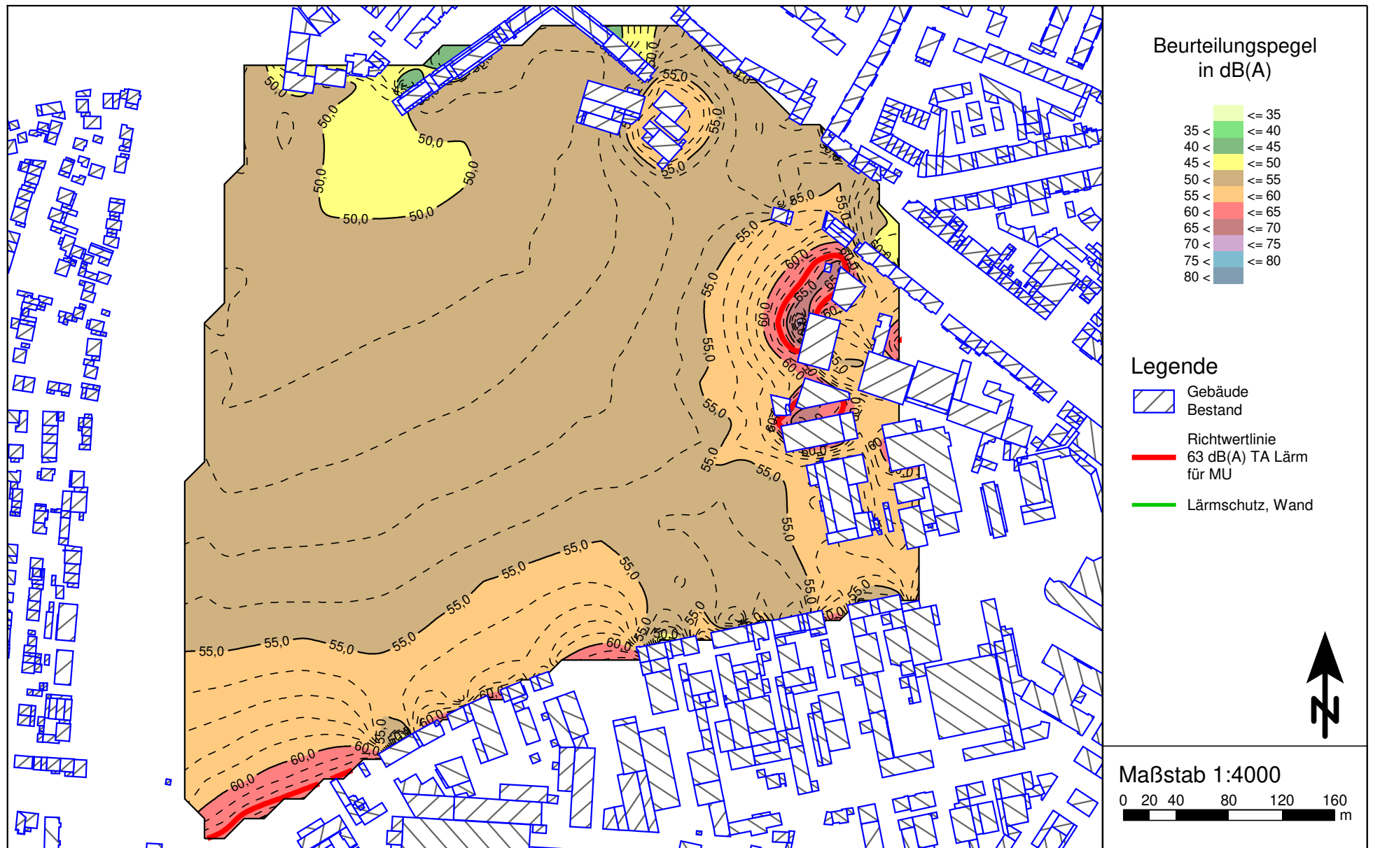
Anlage 26: Ergebnisse der Gewerbelärberechnung bei freier Schallausbreitung in Form einer Isophonenkarte in Höhe von 8 m über Gelände (2. OG.); Tageszeitraum; ohne Berücksichtigung von Ruhezeitenzuschlägen gemäß TA Lärm (z. B. MI oder MU)
