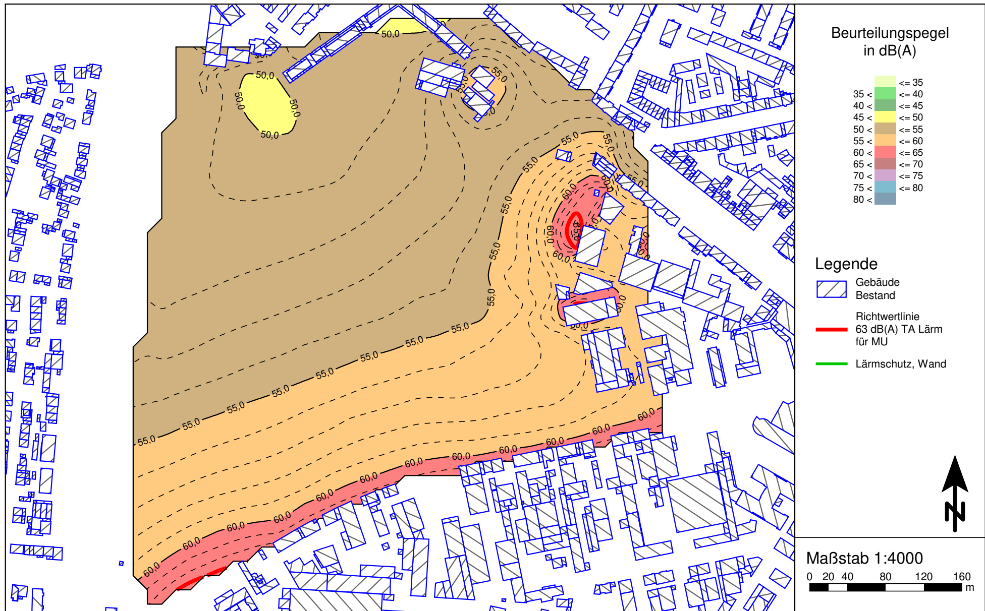
Anlage 28: Ergebnisse der Gewerbelärberechnung bei freier Schallausbreitung in Form einer Isophonenkarte in Höhe von 20 m über Gelände (6. OG.); Tageszeitraum; ohne Berücksichtigung von Ruhezeitenzuschlägen gemäß TA Lärm (z. B. MI oder MU)
