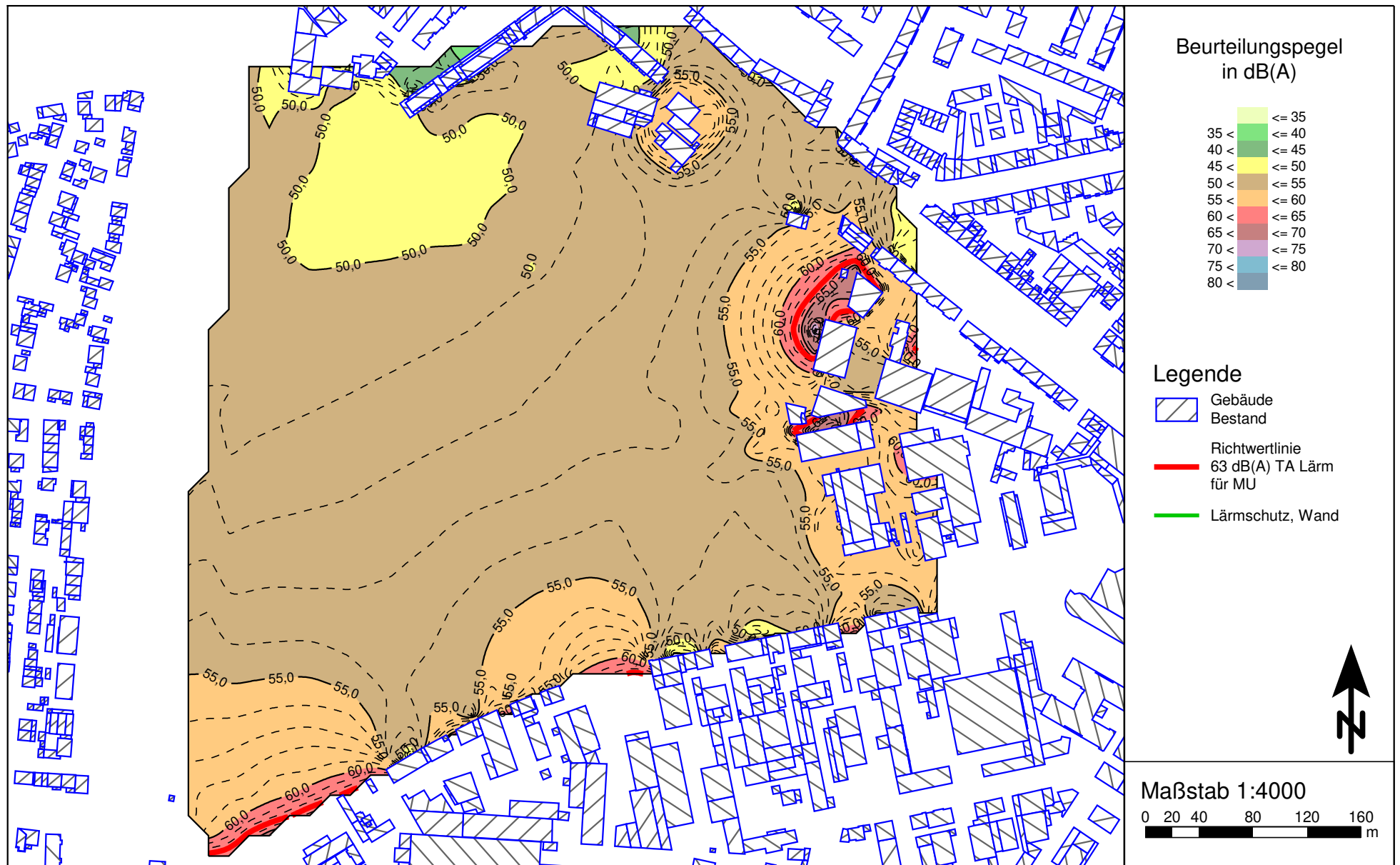
Anlage 24: Ergebnisse der Gewerbelärberechnung bei freier Schallausbreitung in Form einer Isophonenkarte in Höhe von 5 m über Gelände (1. OG.); Tageszeitraum; ohne Berücksichtigung von Ruhezeitenzuschlägen gemäß TA Lärm (z. B. MI oder MU)
