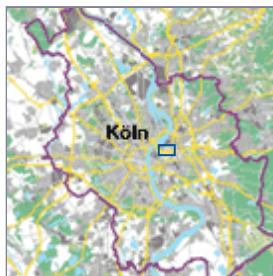
Starkregengefährdung 100-jährliches Ereignis (SRI 7)
